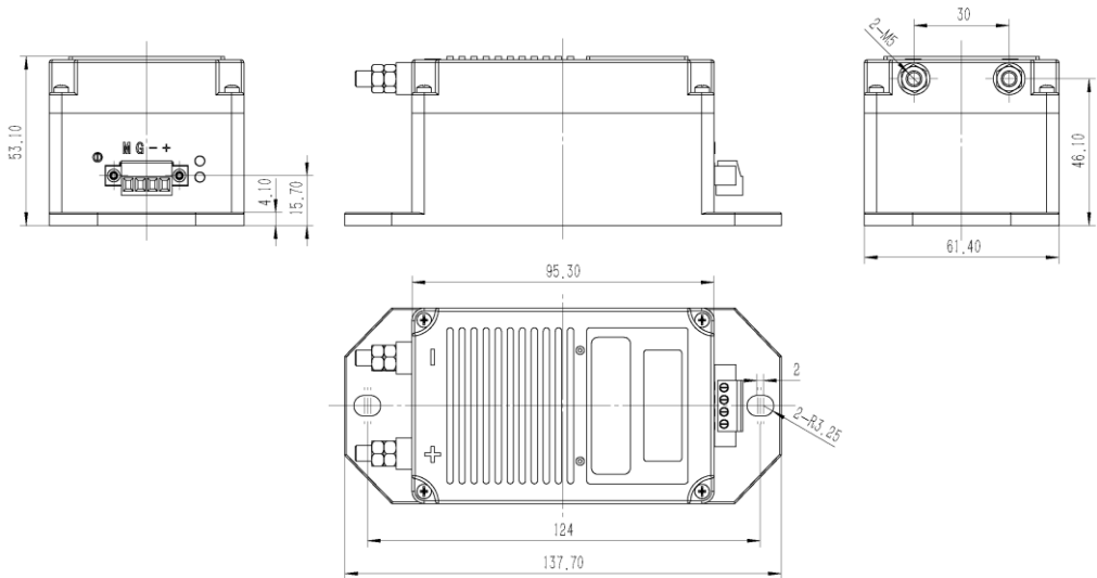
图 1 外形尺寸图
