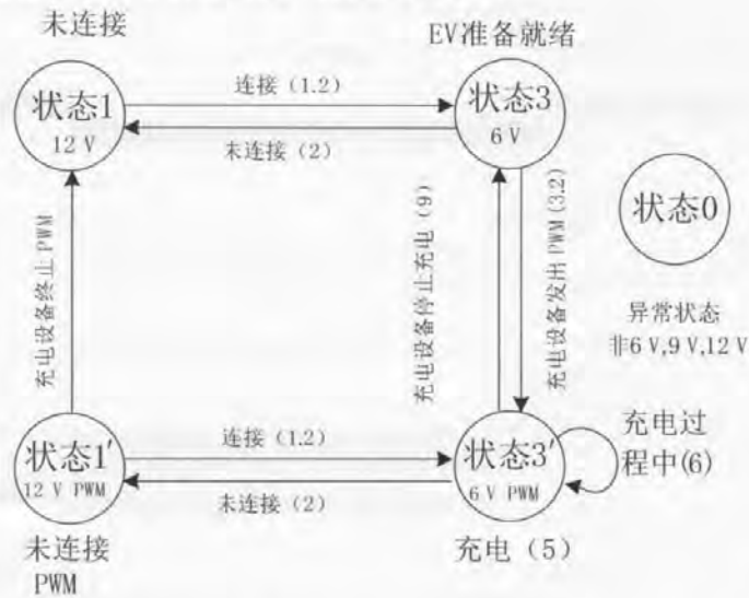
图 A.9 无开关 S2 的交流充电控制导引电路状态转换图
