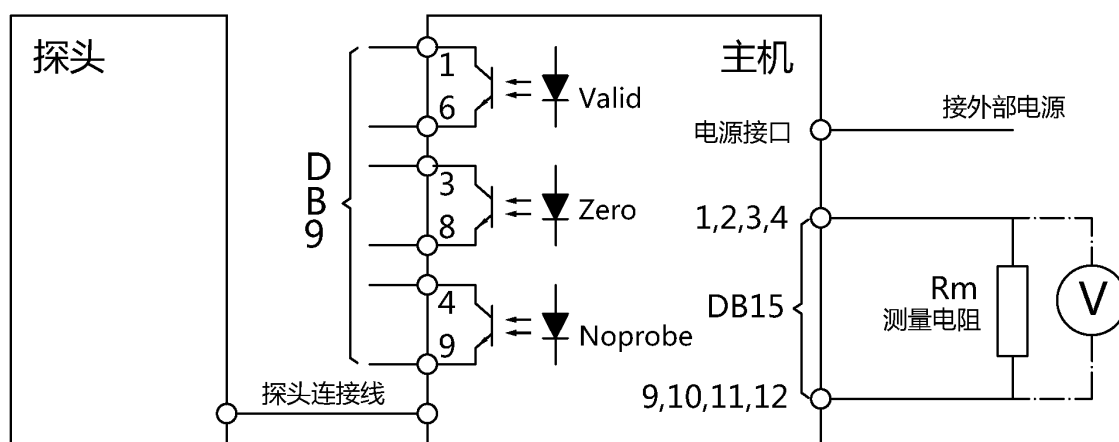
电气连接图
