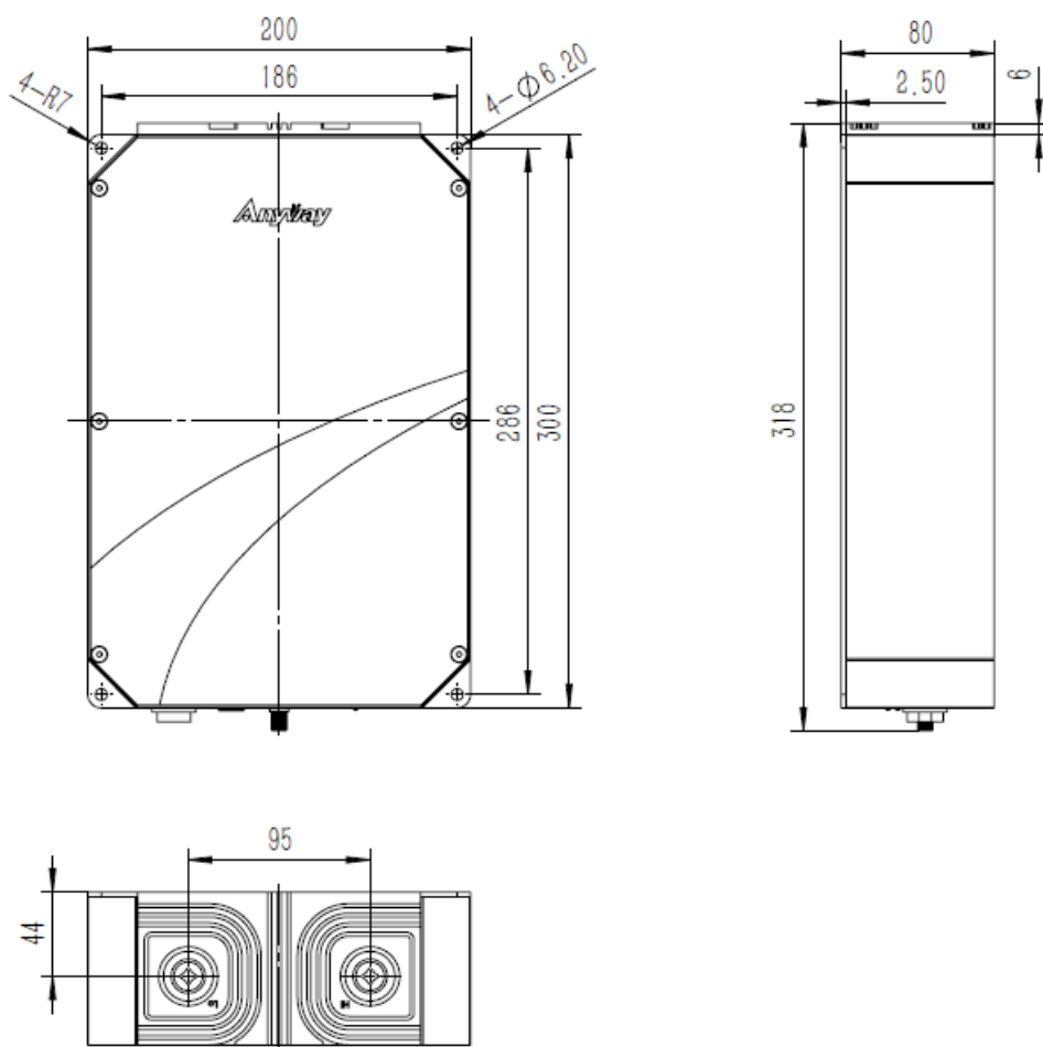
图 1 外形尺寸图
