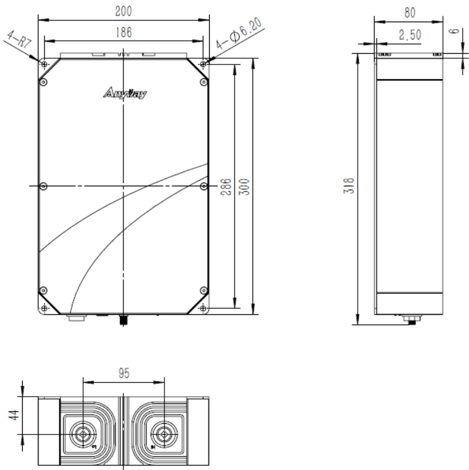
图 1 外形尺寸图
