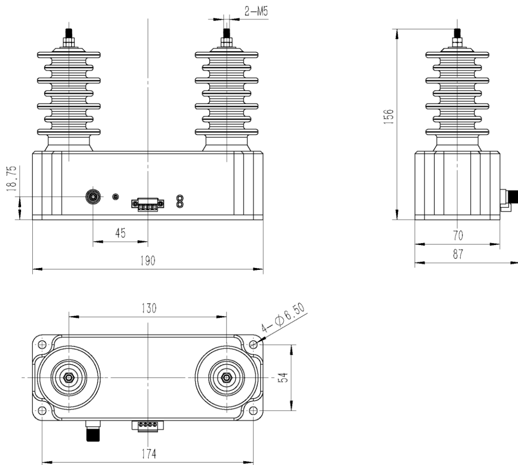
图 1 外形尺寸图
