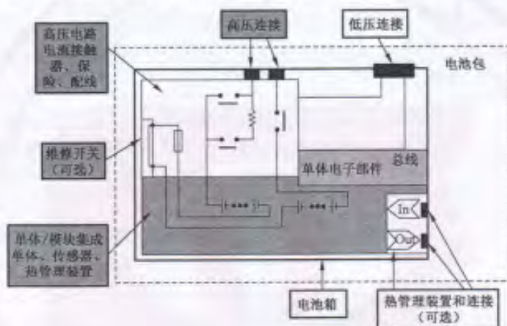
图 A.1 蓄电池包典型结构
