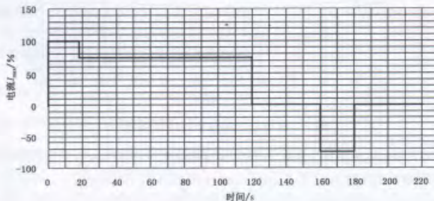
图 1 脉冲功率特性曲线-电流示例
